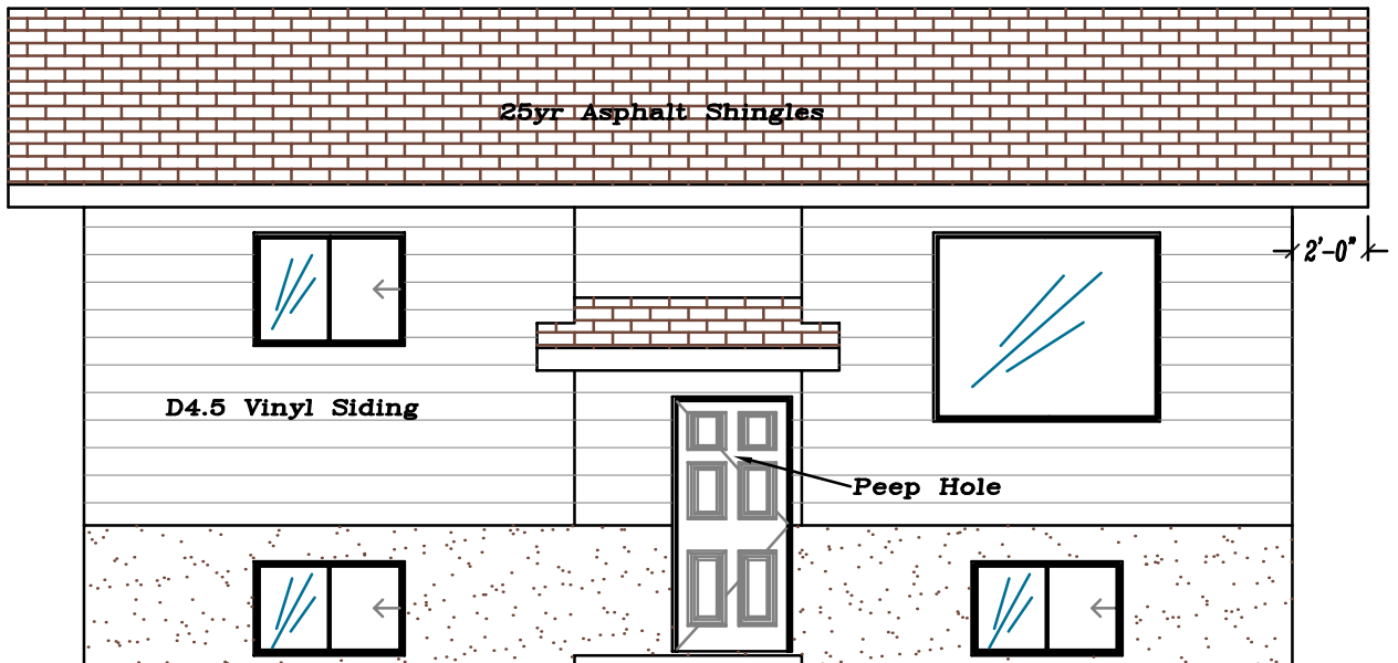
E1 Front Elevation N.T.S.
