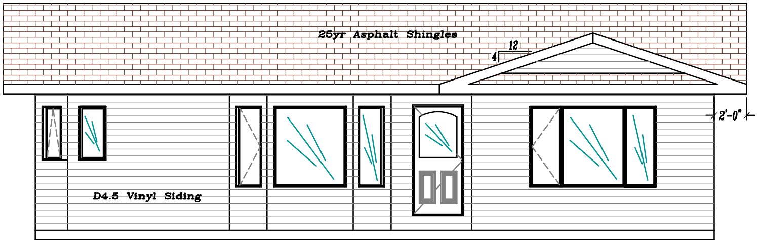
E1 Front Elevation N.T.S.
