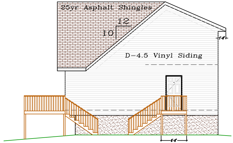
E2 Right Elevation N.T.S.
