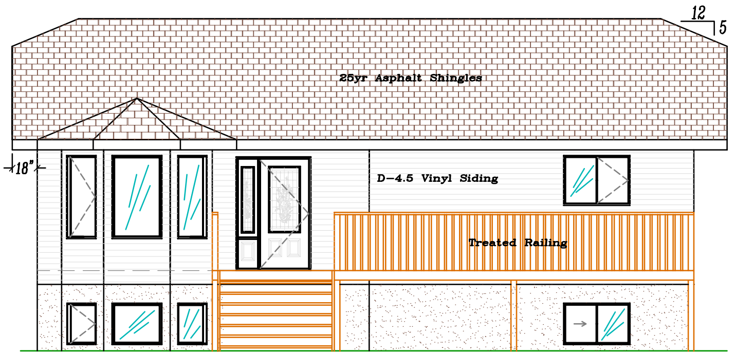
E1 Front Elevation N.T.S.
