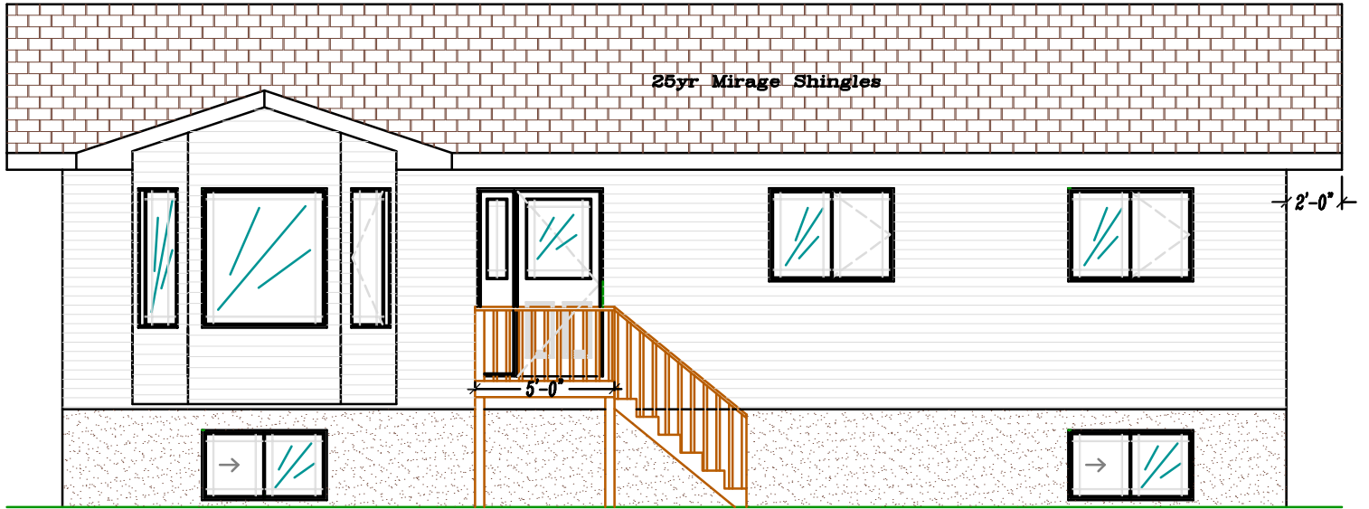
E1 Front Elevation N.T.S.
