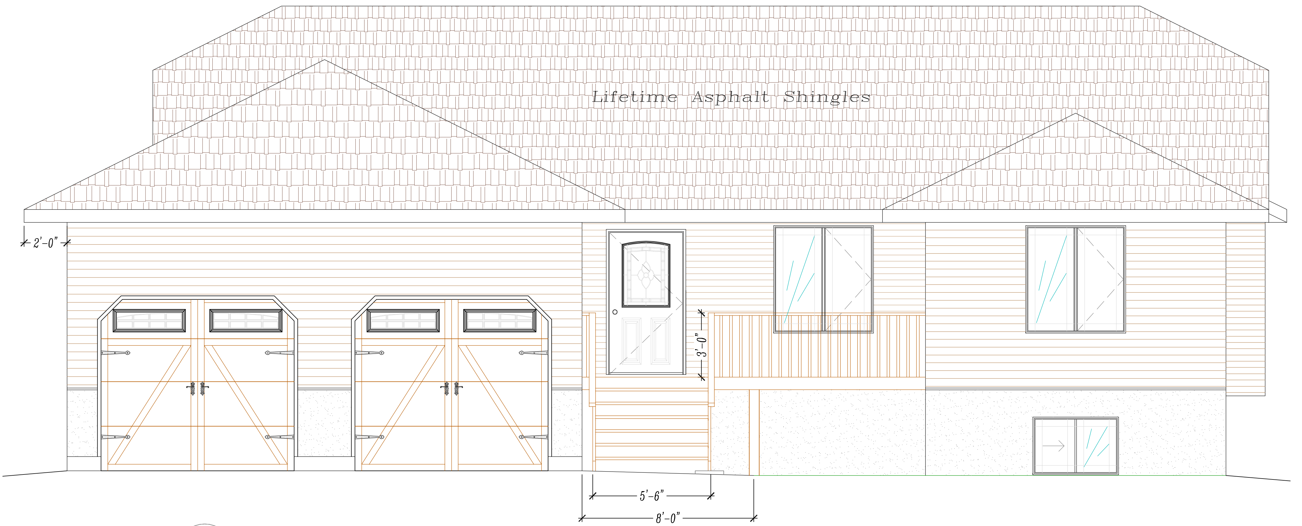
E1 Front Elevation N.T.S.
