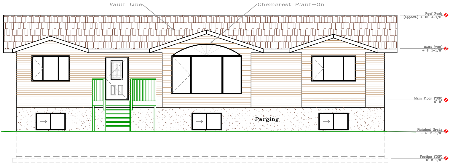
E1 Front Elevation N.T.S.
